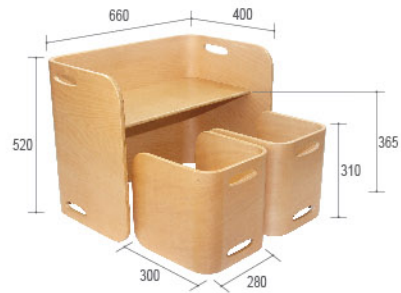
原木色 Natural
